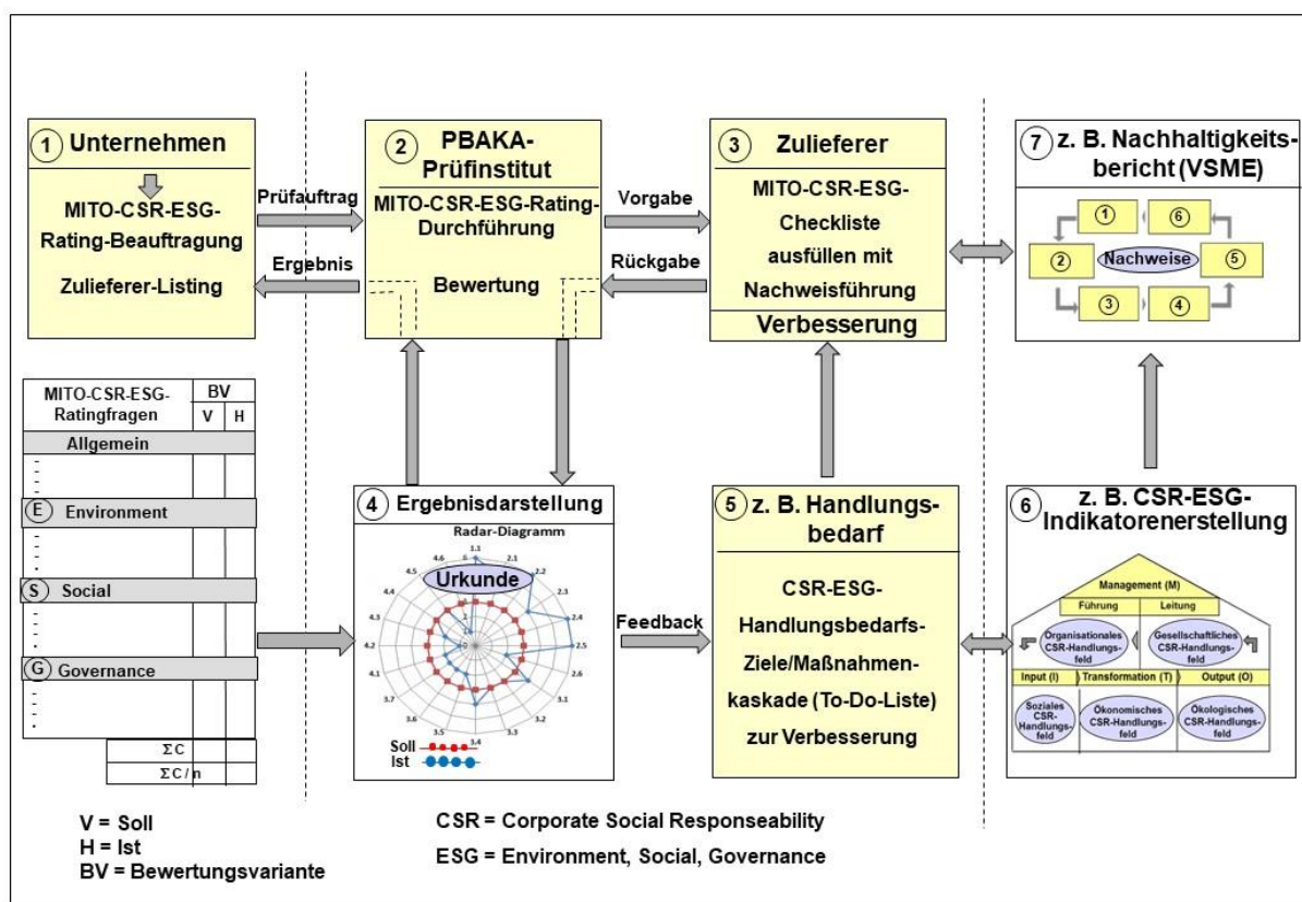
Abbildung 1: MITO-CSR-ESG-Rating-Vorgehensmodell
