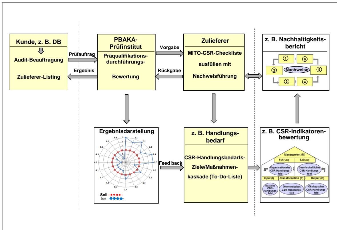
Abbildung 1: MITO-modellbezogenes CSR-Präqualifikations-Vorgehensmodell
