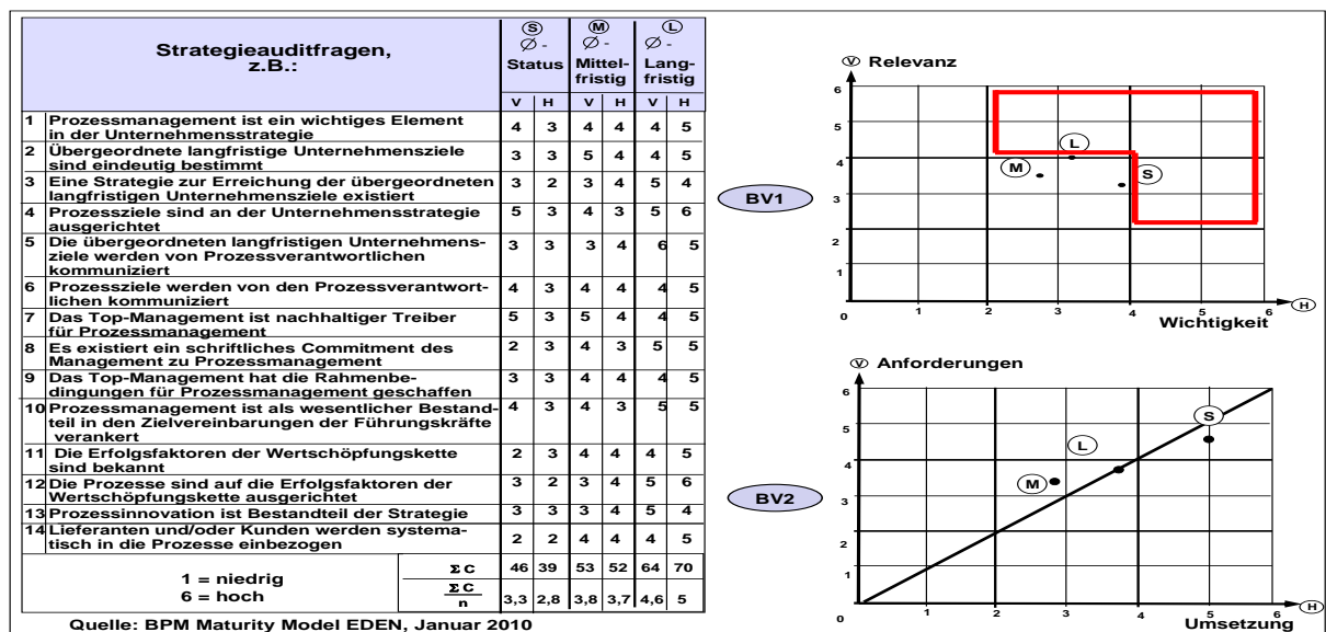
Abbildung 1: Prozessmanagementbezogenes Strategieumsetzungsaudit
